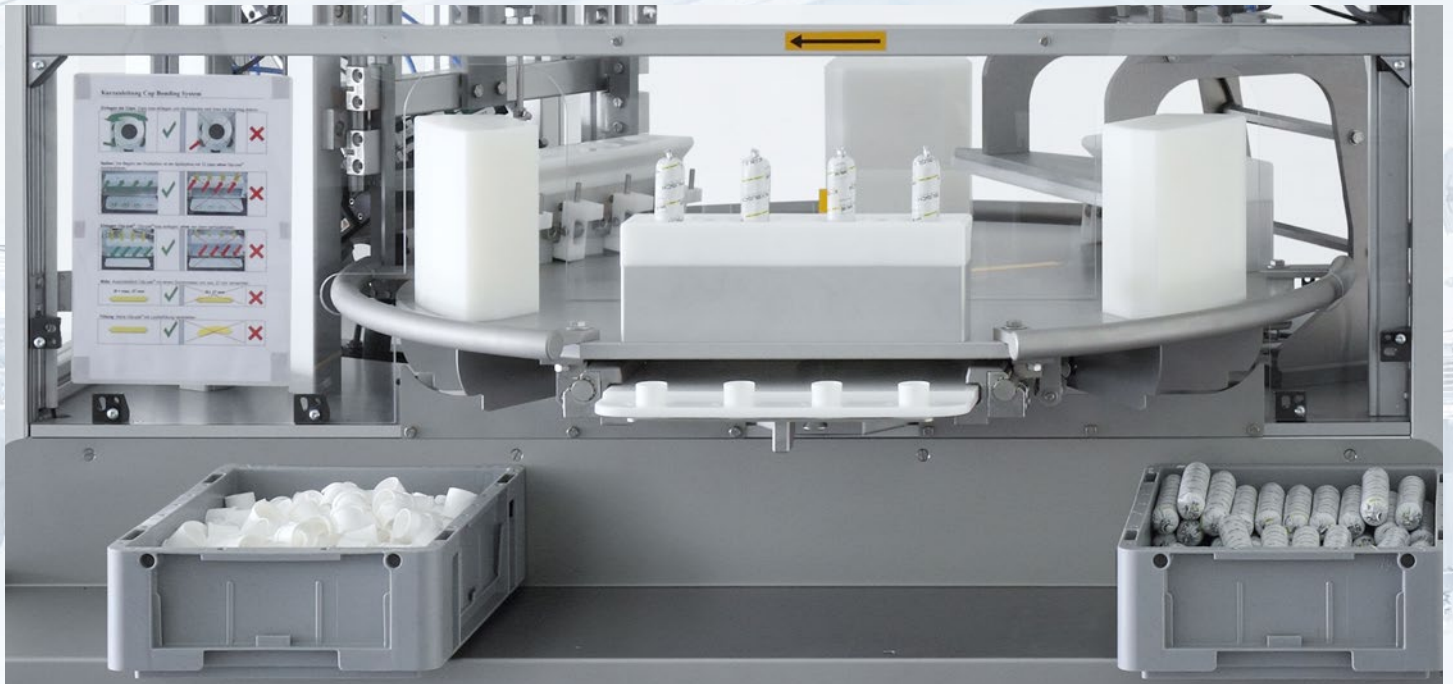
Drehteller mit vier Aufnahmen für clip-pak®
