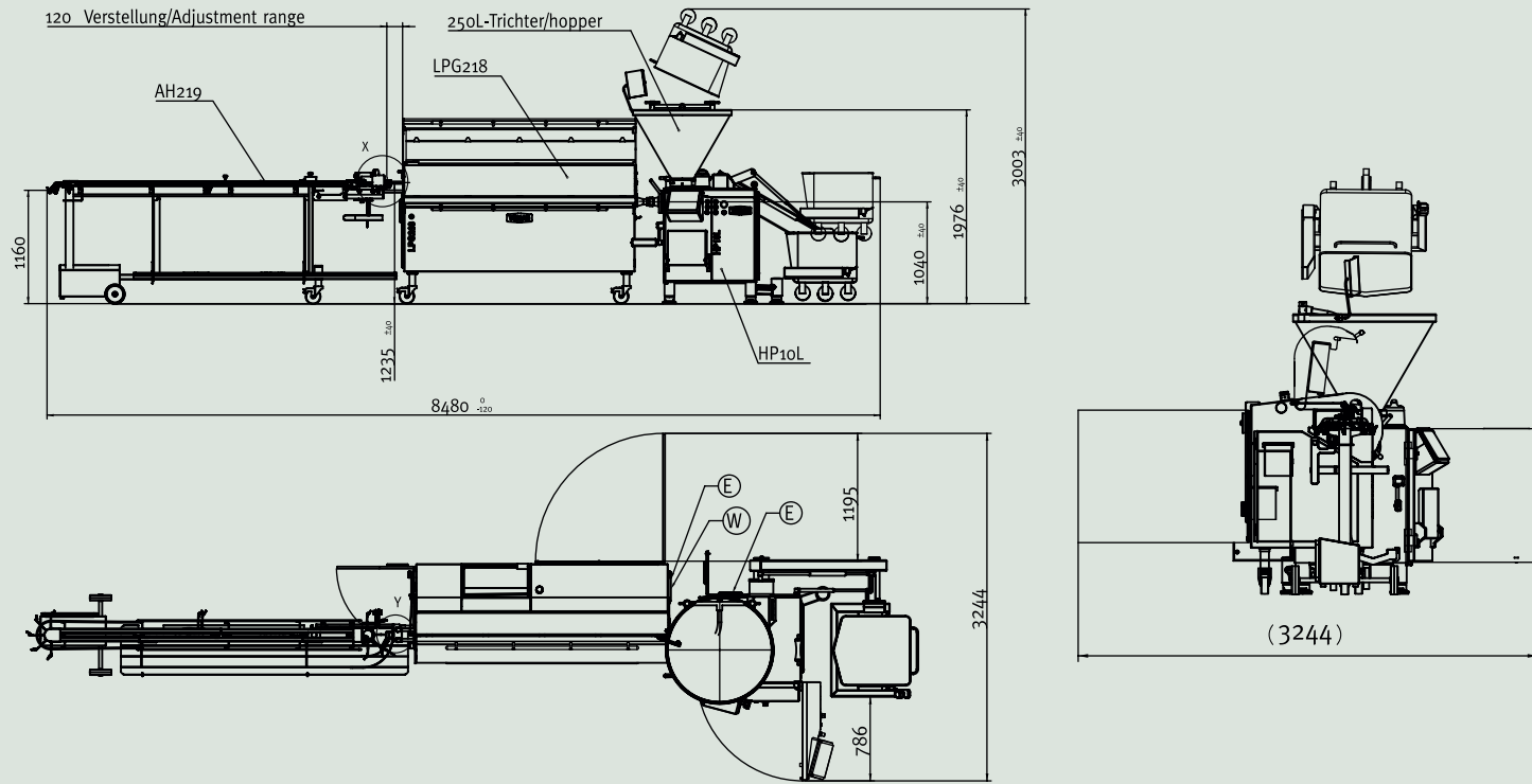
Technische Zeichnung
